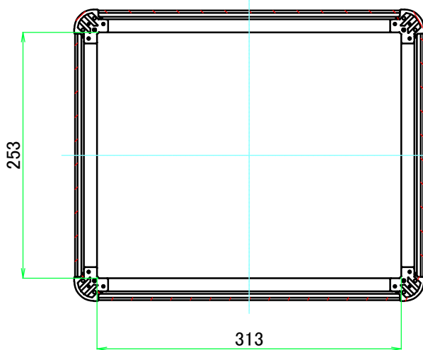
C-C ( 1 : 5.5 )
