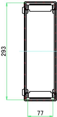
A-A ( 1 : 5.5 )
