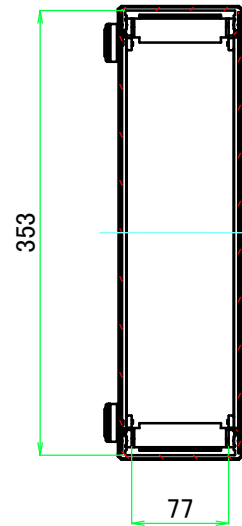
A-A (1:6)
