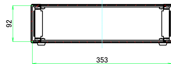
B-B ( 1 : 5.5 )
