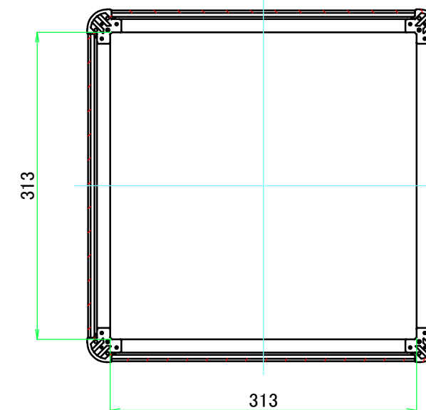
C-C ( 1 : 5.5 )
