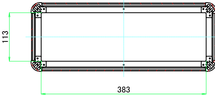
C-C ( 1 : 5.5 )
