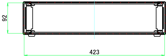
B-B ( 1 : 5.5 )
