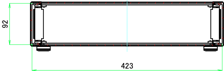
B-B ( 1 : 5 )
