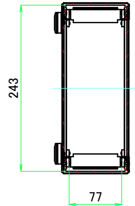
A-A ( 1 : 5.5 )
