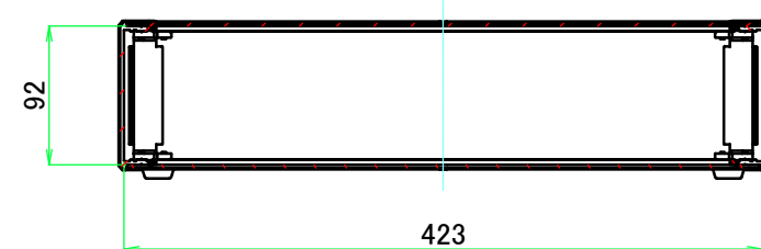
B-B ( 1 : 5.5 )
