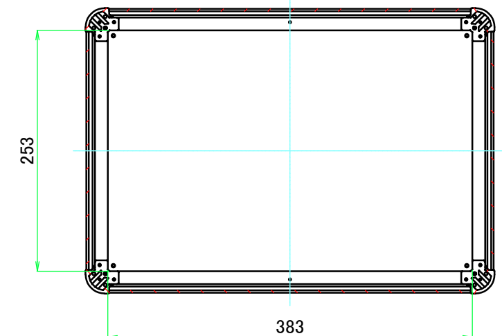
C-C ( 1 : 5.5 )
