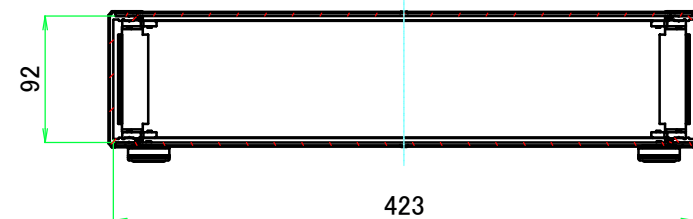
B-B ( 1 : 5.5 )
