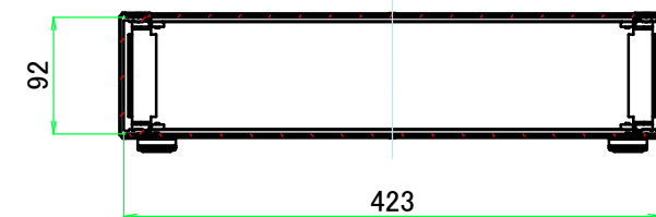
B-B ( 1 : 6.5 )
