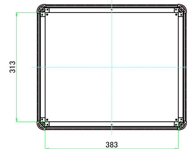
C-C ( 1 : 6.5 )
