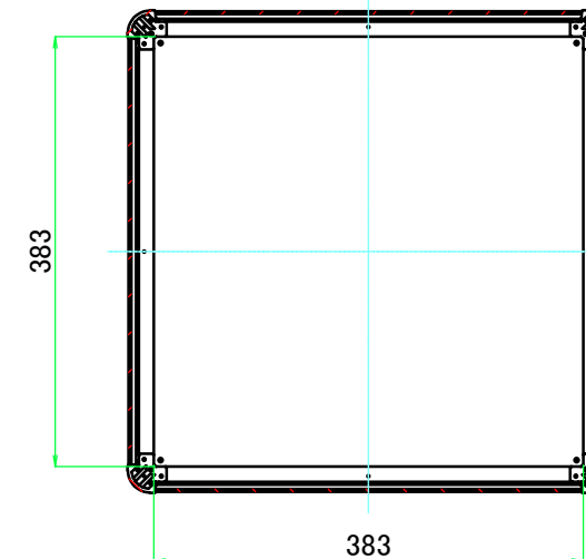
C-C ( 1 : 7.5 )
