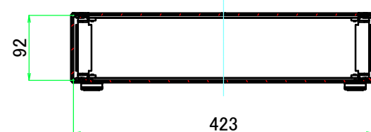
B-B ( 1 : 7.5 )
