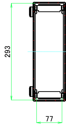
A-A ( 1 : 6.5 )
