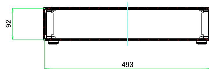
B-B ( 1 : 6.5 )
