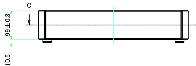
B-B ( 1 : 6.5 )
