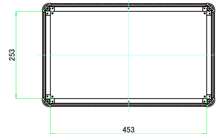
C-C ( 1 : 6.5 )
