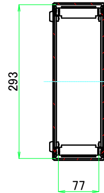
A-A (1:7)
