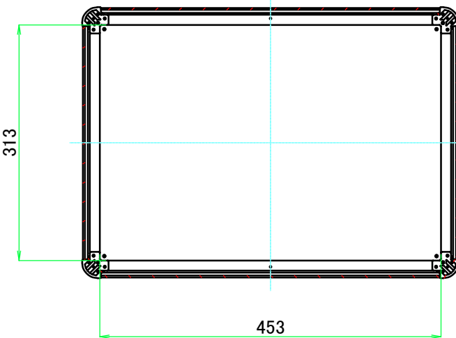
C-C ( 1 : 7 )
