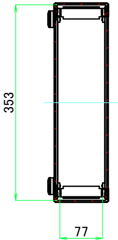
A-A ( 1 : 7 )
