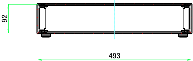
B-B ( 1 : 7 )
