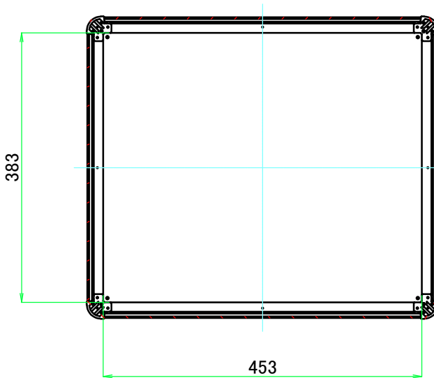
C-C ( 1 : 7.5 )
