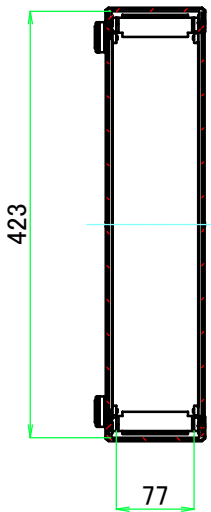
A-A ( 1 : 7.5 )
