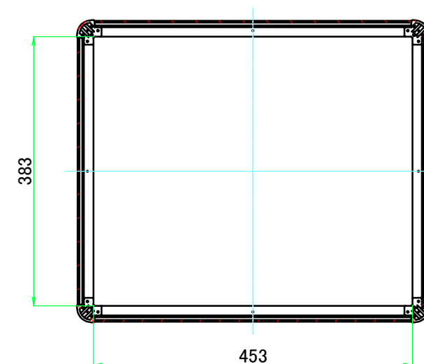
C-C ( 1 : 7.5 )
