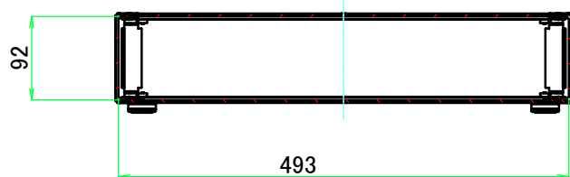
B-B ( 1 : 7.5 )
