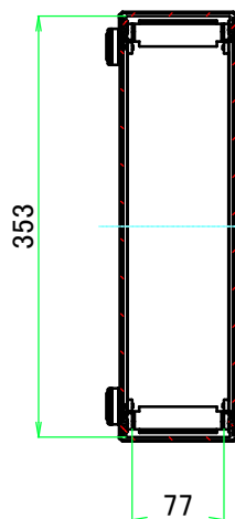
A-A (1:7)
