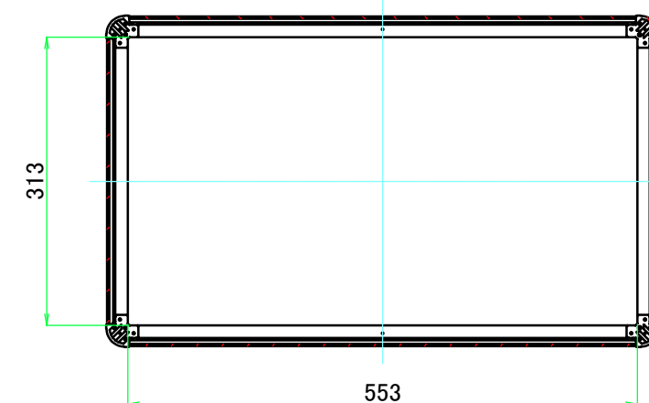
C-C ( 1 : 7.5 )
