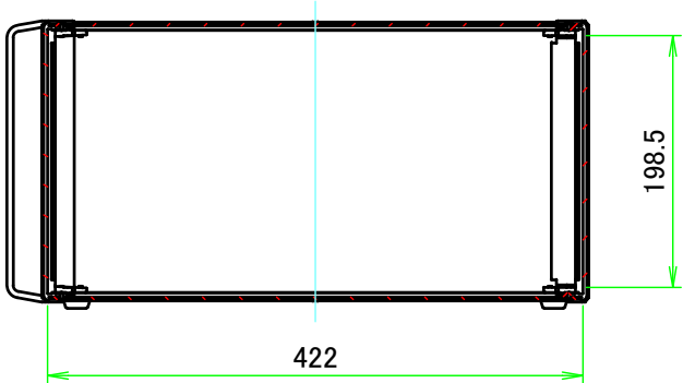
A-A (1:6.5)
