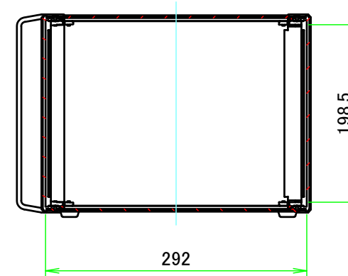
A-A (1:6)
