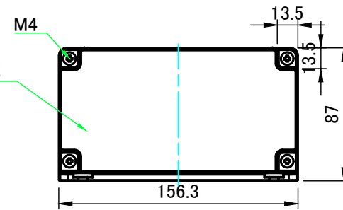
A-A (1:3.5)
