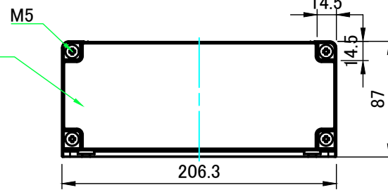
フランジ付側板2 Flanged end panel 2
