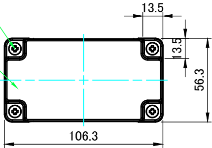
パネル2 End panel 2
