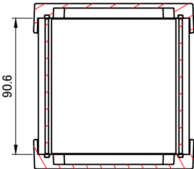
C-C ( 1 : 2.5 )
