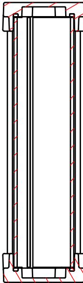
B-B ( 1 : 2.5 )
