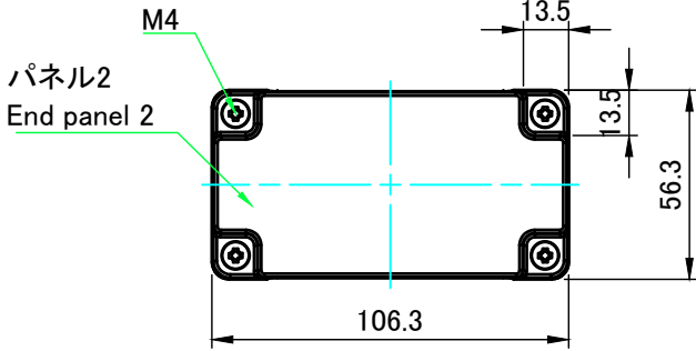
A-A ( 1 : 2.5 )
