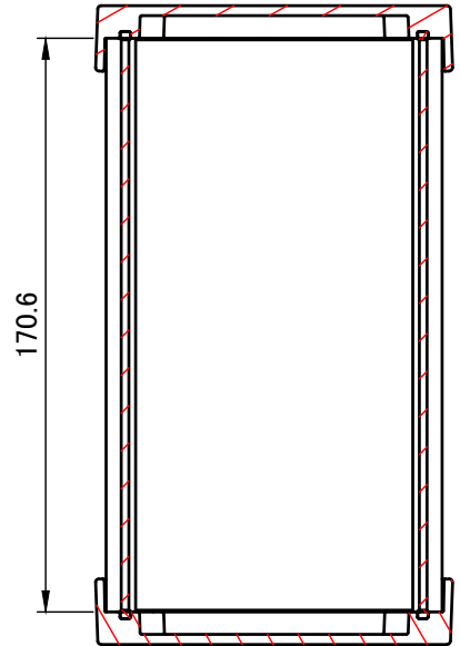
C-C ( 1 : 2.5 )
