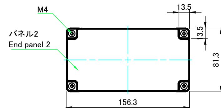
A-A (1:3)
