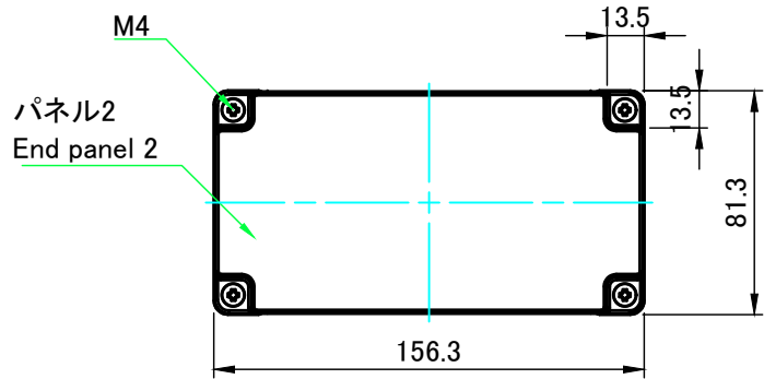
A-A (1:3)
