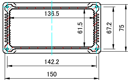
A-A (1:3)
