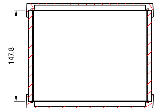
C-C ( 1 : 3.5 )
