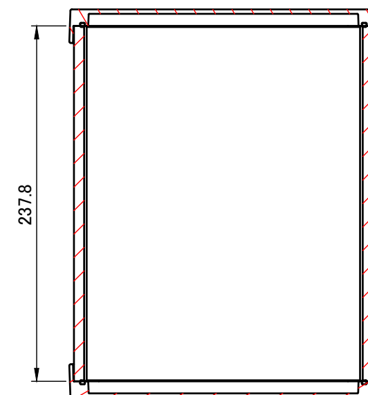
C-C ( 1 : 3.5 )
