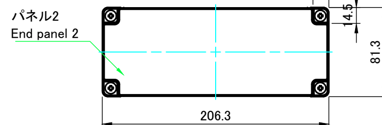
A-A (1:3.5)
