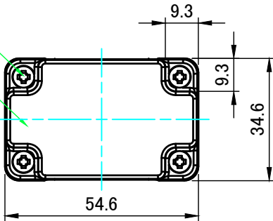
A-A ( 1 : 1.5 )
