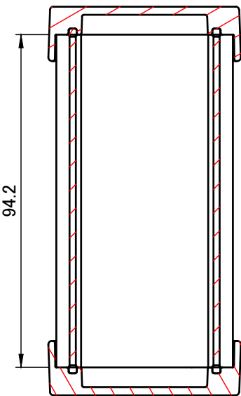
C-C ( 1 : 1.5 )
