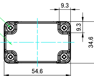
A-A ( 1 : 1.5 )
