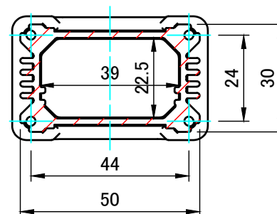
A-A ( 1 : 1.5 )
