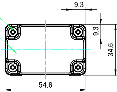
A-A ( 1 : 1.5 )
