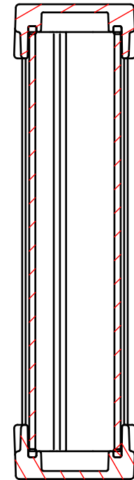
B-B ( 1 : 1.5 )
