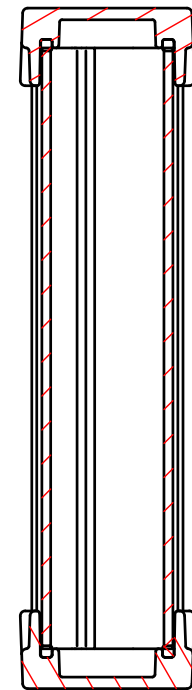
B-B ( 1 : 1.5 )
