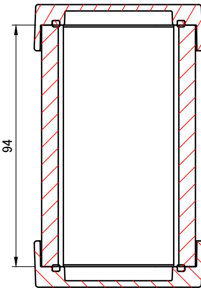
C-C ( 1 : 1.5 )
