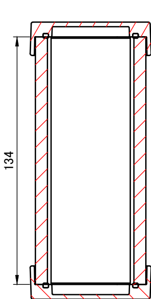
C-C ( 1 : 2 )
