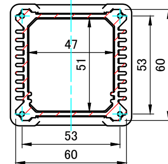
A-A (1:2)
