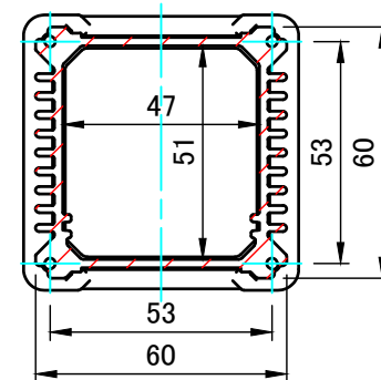
A-A (1:2)
