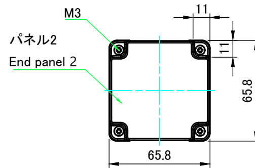
A-A ( 1 : 2.5 )
