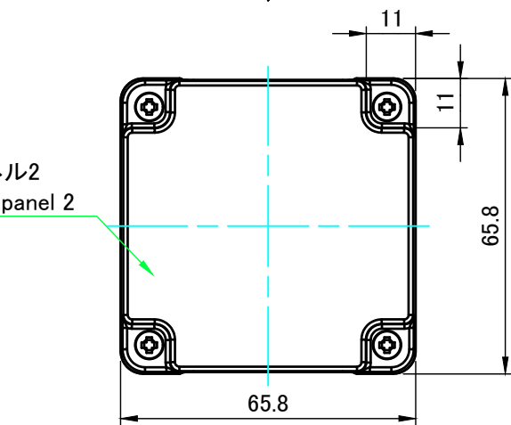
A-A ( 1 : 1.5 )
