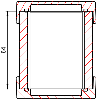
C-C ( 1 : 1.5 )
