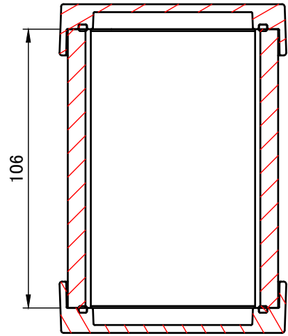
C-C (1:2)
