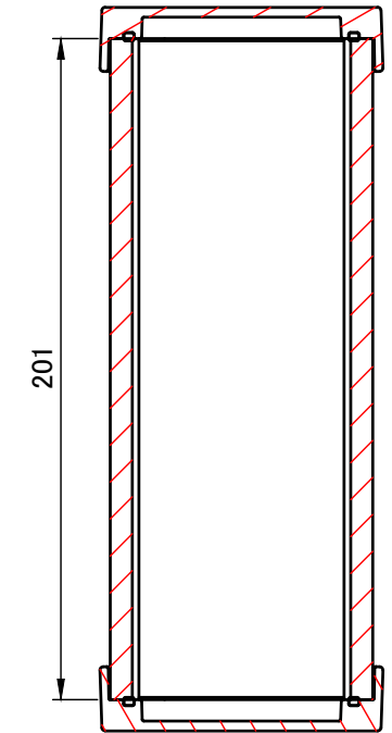
C-C ( 1 : 2.5 )
