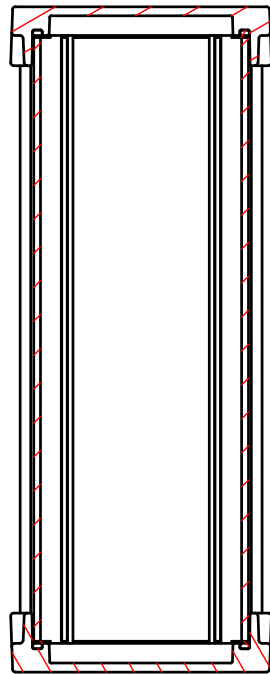
B-B ( 1 : 2.5 )
