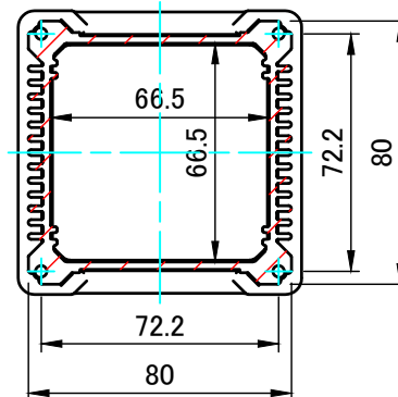
A-A ( 1 : 2.5 )
