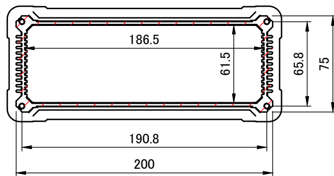
A-A (1:3)
