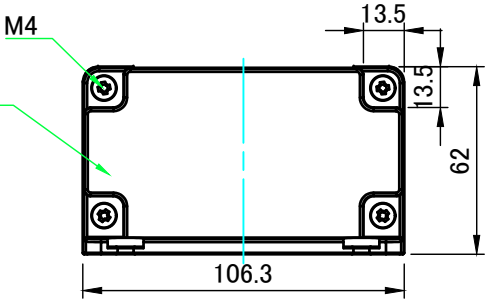
A-A ( 1 : 2.5 )
