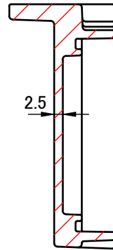
B-B ( 1 : 1.5 )
