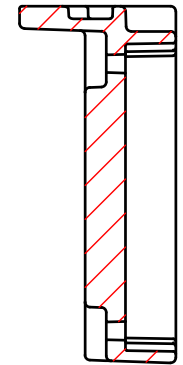
D-D ( 1 : 1.5 )
