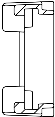
A-A断面図
