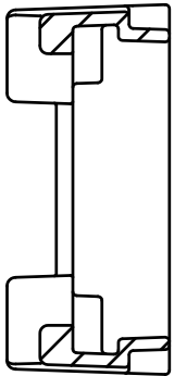
A-A断面図
