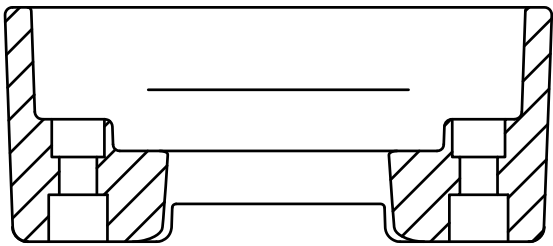
B-B断面図
