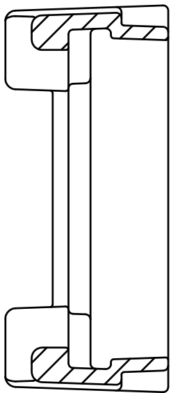
A-A断面図
