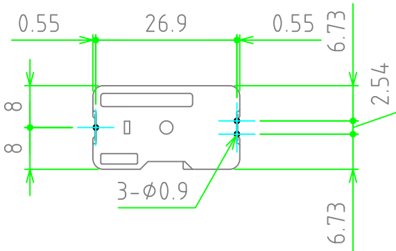
取付穴寸法
