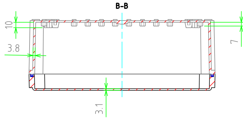
ボディ(内視)
