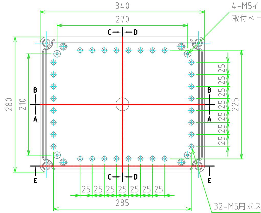
ボディ(内視)
