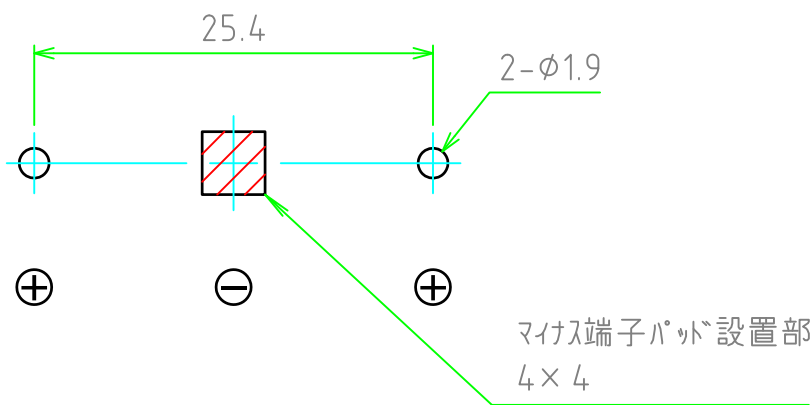
基板実装図
